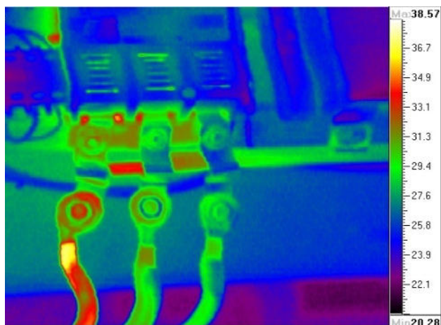
Рисунок 21. Пример термограммы контактных соединений с температурной шкалой
